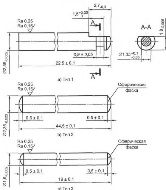
Рисунок 2 – Контрольные оправки
