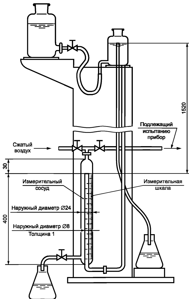
Рисунок 1 — Устройство для испытания аппарата на герметичность
