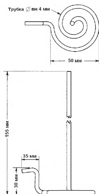
Рисунок 1 – Подающая трубка
