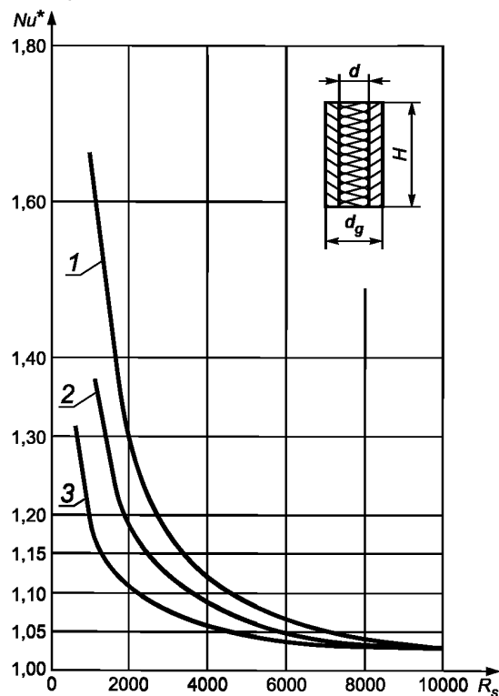
Рисунок А.4 — Диаграмма для теплоизоляционной системы общей толщиной d_g = 0,20 \text{ м}
