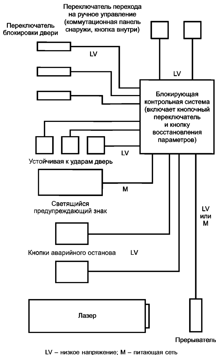
Рисунок А.3 — Система блокировки с запиранием
