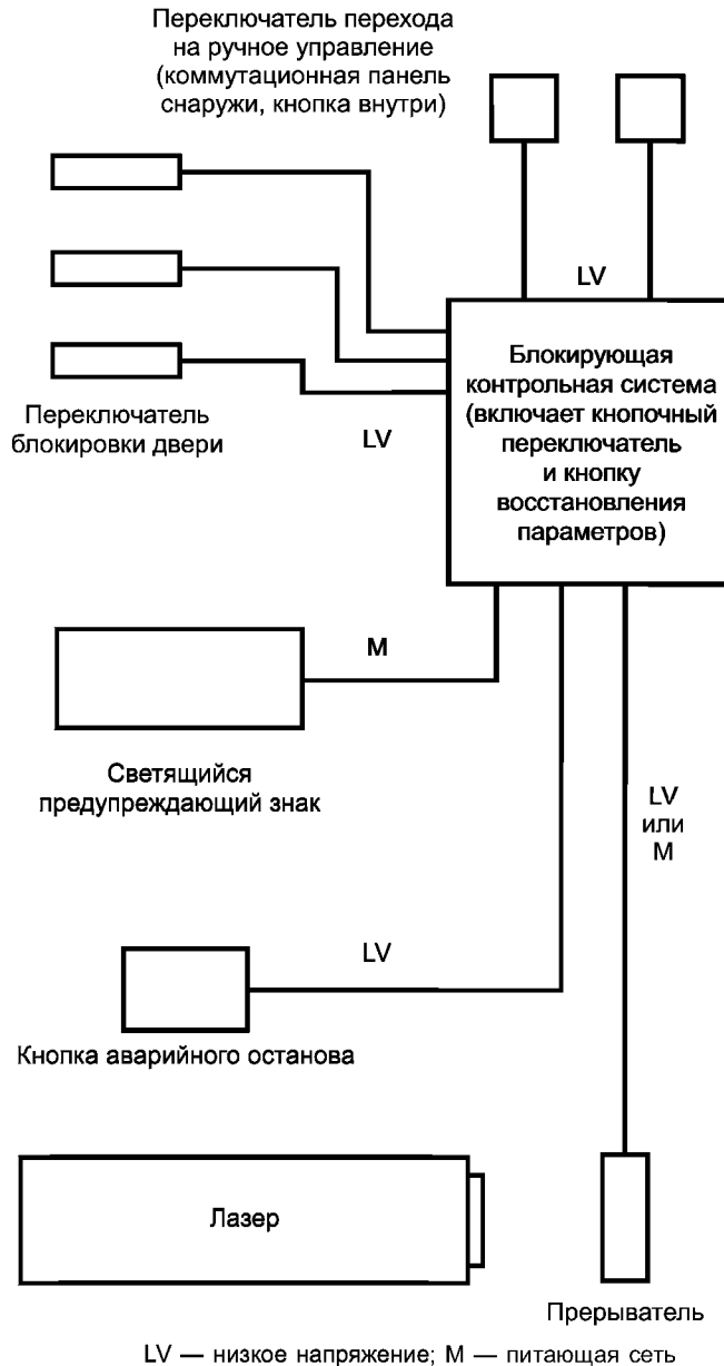
Рисунок A.2 — Система блокировки без запирания
