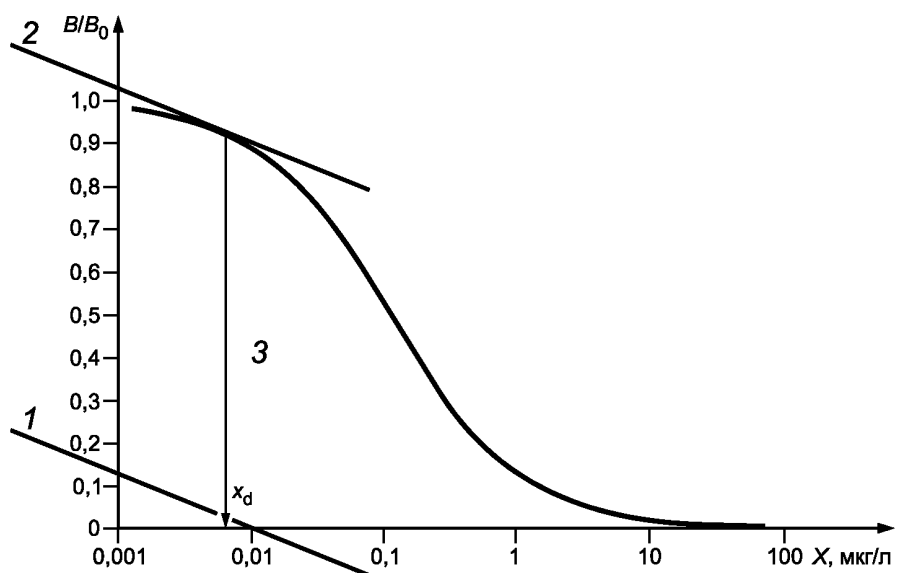
Рисунок 6 — Полулогарифмический график кривой B/B_0 для конкурентного иммуноферментного анализа ELISA 17-гидроксиprogестерона
