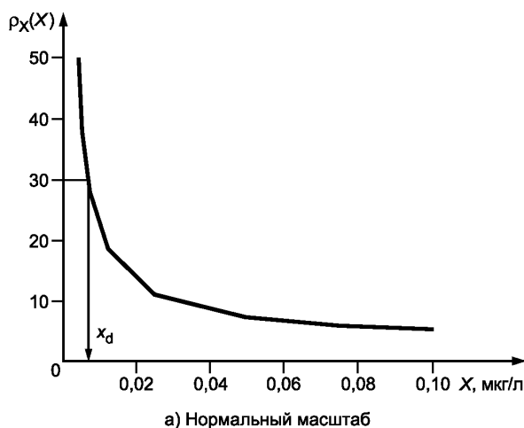
Рисунок 5 — Коэффициент вариации приведенной переменной состояния \rho_X(X) (функция прецизионности) и минимальное обнаруживаемое значение x_d в нормальном и полулогарифмическом масштабе для конкурентного иммуноферментного анализа ELISA (Лист 1)
