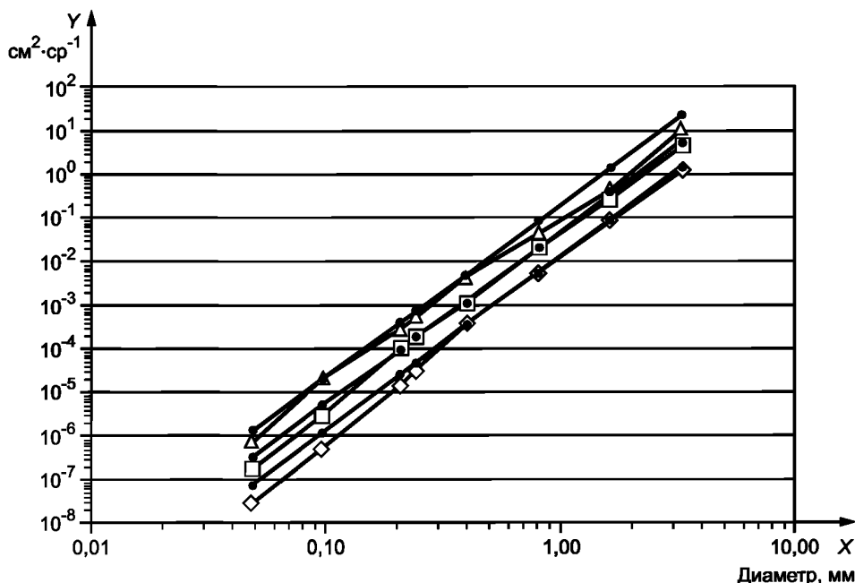
Рисунок В.4 — Зависимость экспериментально полученных значений площади поперечного сечения обратного рассеяния от плоского торца проволочек из нержавеющей стали от их диаметра на частотах 9,6 МГц ( \Delta ), 4,8 МГц ( \square ) и 2,4 МГц ( \diamond ) [29]
