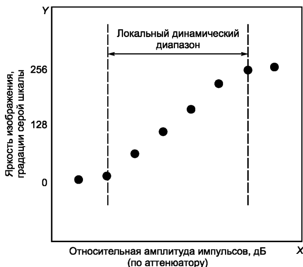
Рисунок 5 — Значения яркости оцифрованного изображения в зависимости от параметров аттенюатора при измерении локального динамического диапазона с помощью внешнего акустического сигнала
