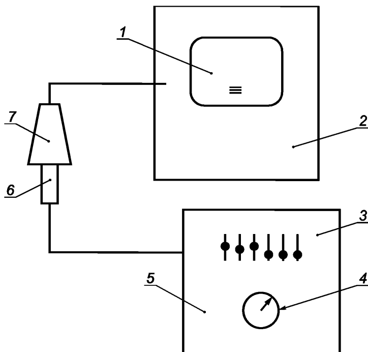
1 — изображение сигнала в В-режиме; 2 — ультразвуковой сканер; 3 — аттенуатор; 4 — задержка импульсов; 5 — генератор тональных импульсов; 6 — излучатель; 7 — датчик сканера
