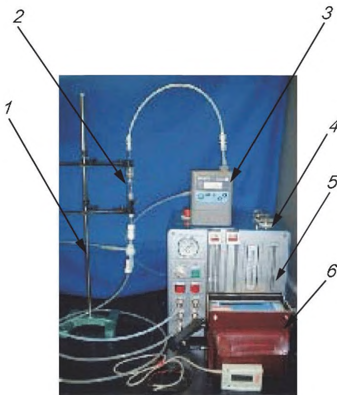
1 — штатив; 2 — трубка для образца экстракционная стеклянная, страна-изготовитель Япония; 3 — мининасос; 4 — мембранный разделитель: PD-1B-2; 5 — детектор Fromtector XP-308B; 6 — регистратор
