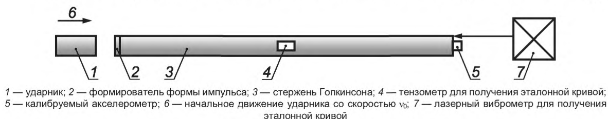
Рисунок 6 — Схема калибратора удара со стержнем Гопкинсона
