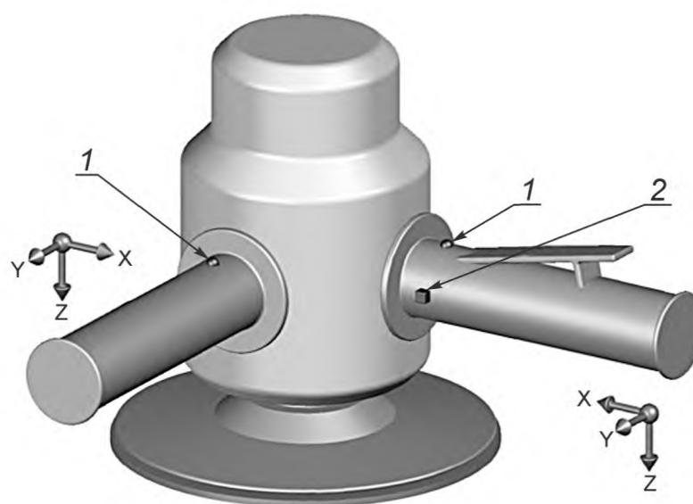
Рисунок 10 — Точки и направления измерений для вертикальной шлифовальной/полировальной машины
