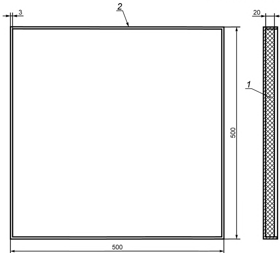
Рисунок С.1 — Поглотитель энергии
