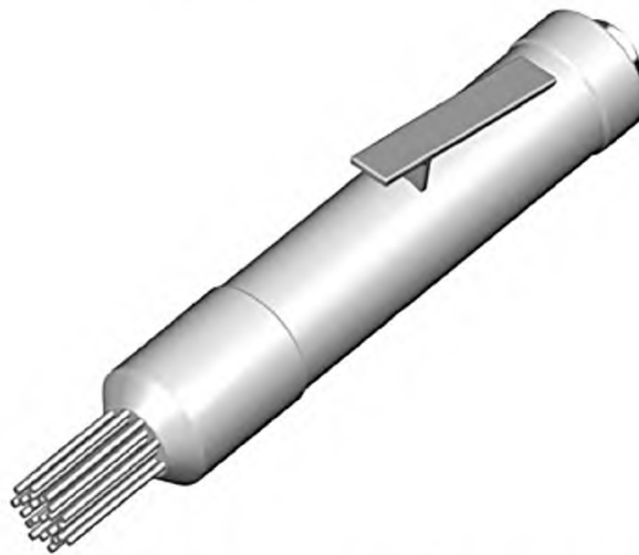
Рисунок 2 — Прямой пучковый зачистной молоток
