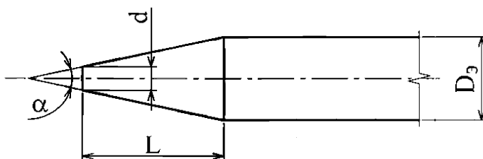
Рисунок 1 – Форма заточки вольфрамового электрода
