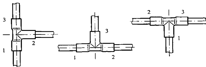
Рисунок 4 – Последовательность пайки соединений тройников в зависимости от пространственного положения
