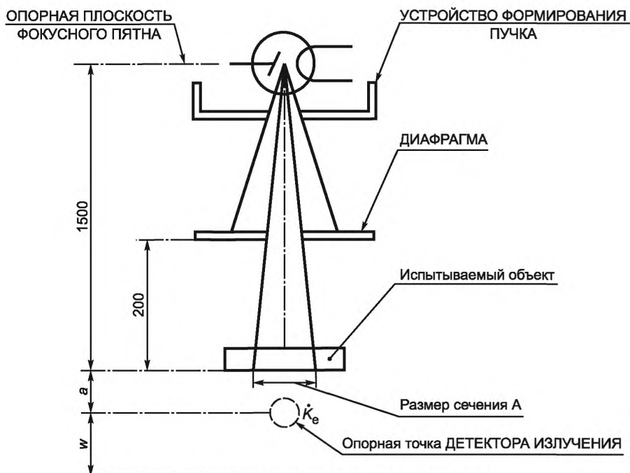
Рисунок 2 — Геометрия УЗКОГО ПУЧКА
