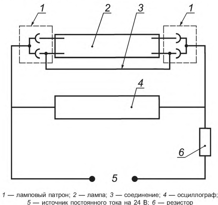
Рисунок 3 — Схема испытания осветительного устройства на вибрацию
