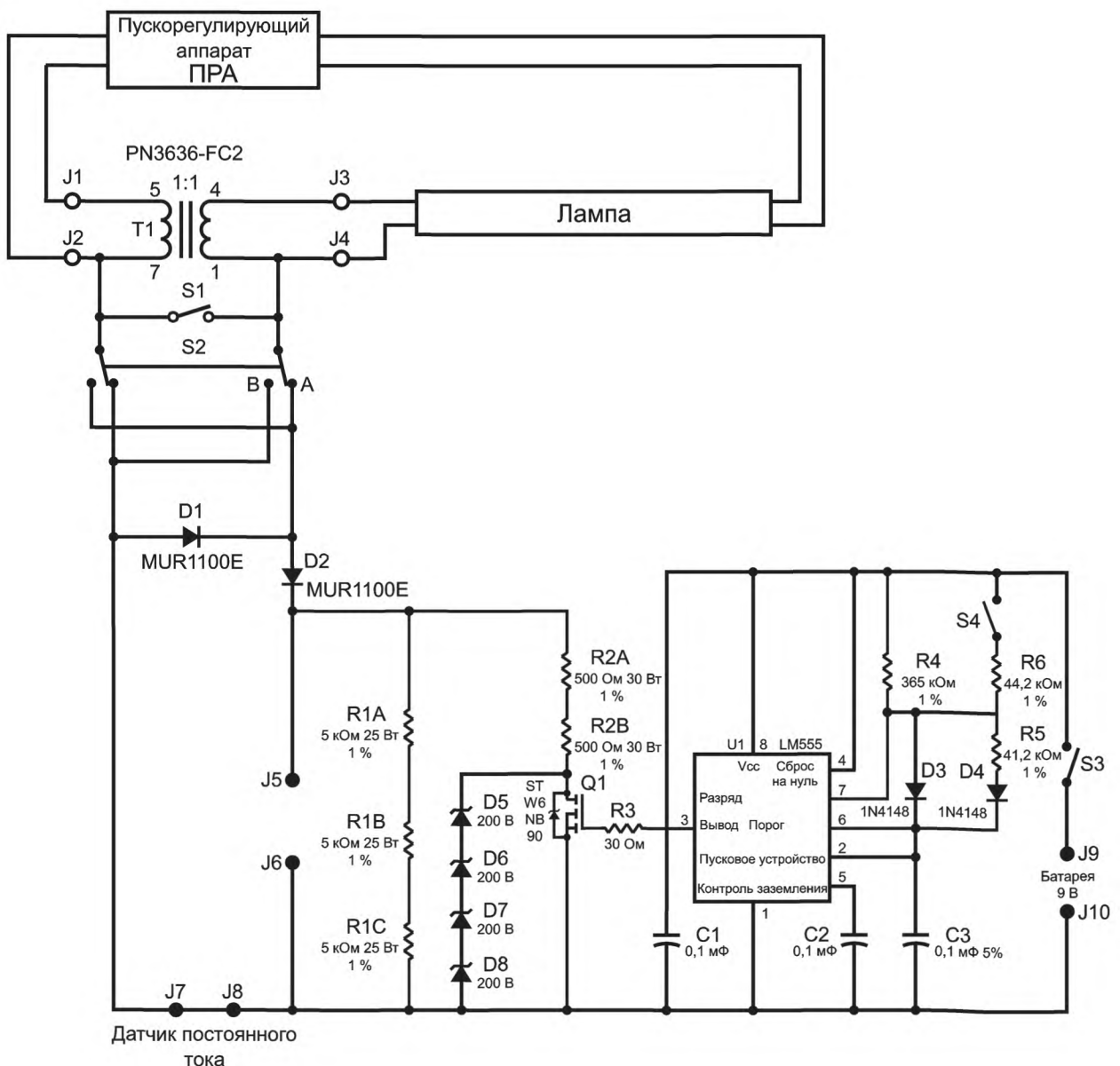
Рисунок Н.1 — Схема испытания асимметричным импульсом
