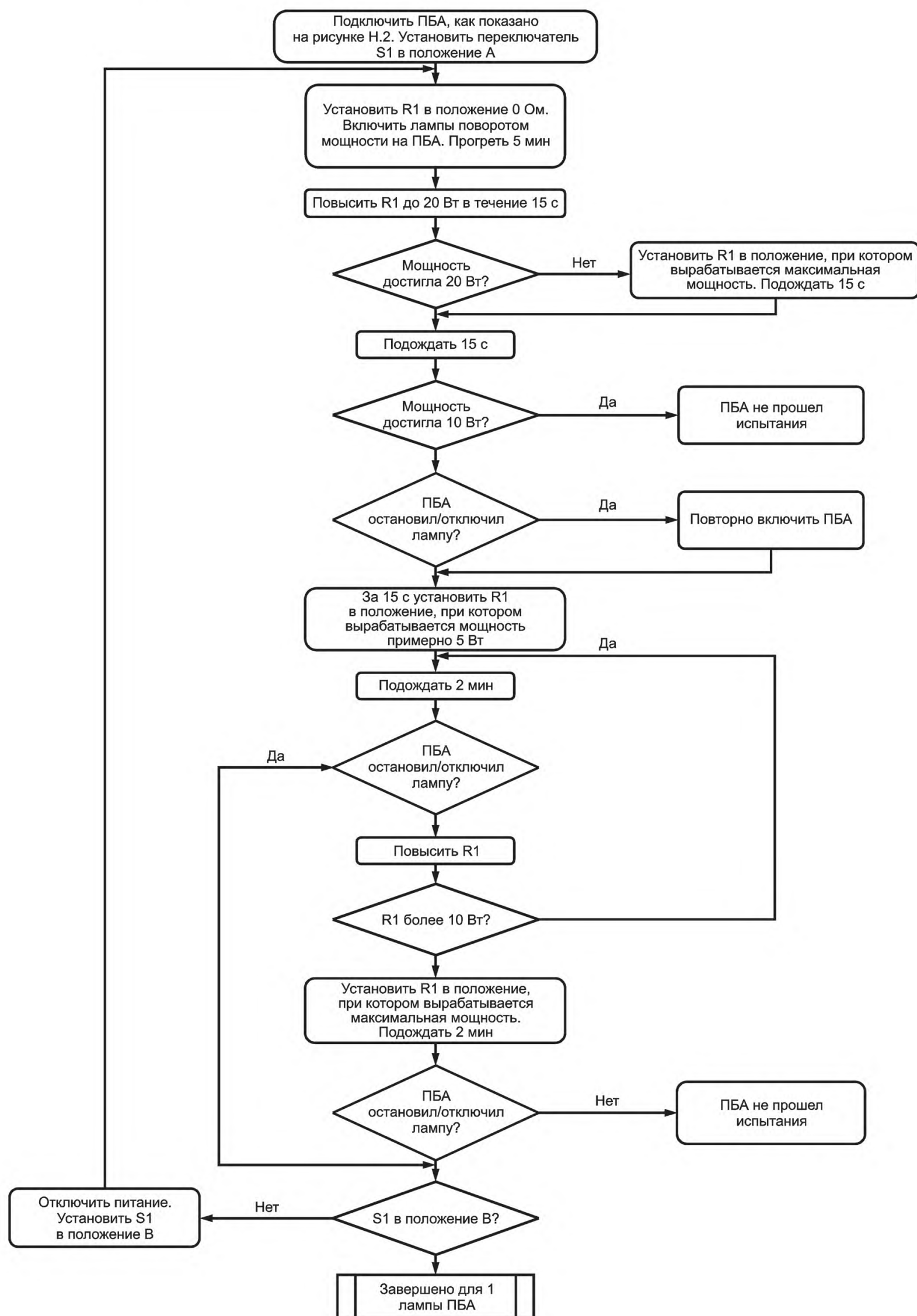
Рисунок Н.3 — Блок-схема испытания асимметричной мощностью
