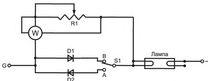
Рисунок Н.2 — Схема испытаний асимметричной мощностью
