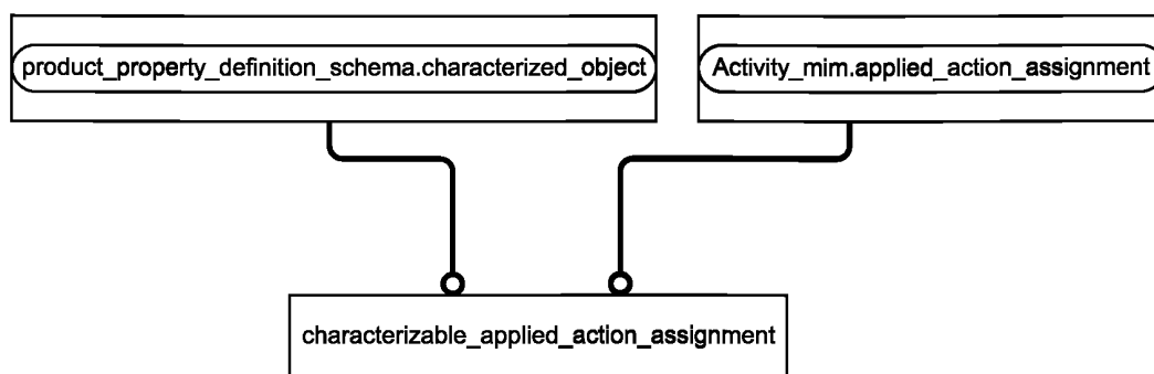
Рисунок D.7 — Представление IMM на уровне объектов в формате EXPRESS-G (диаграмма 6 из 6)
