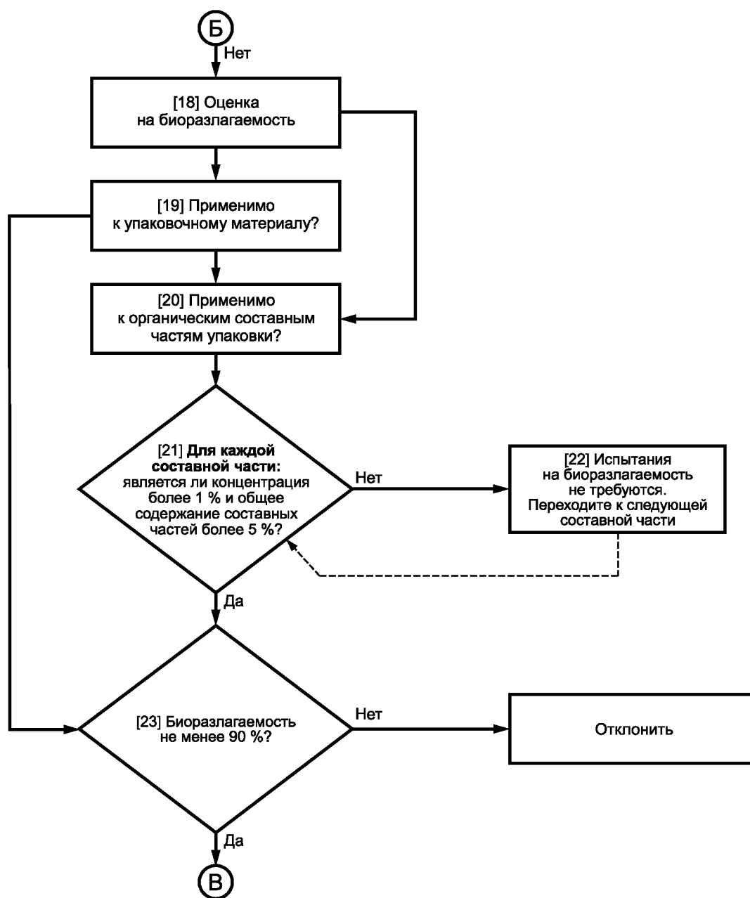
Рисунок В.1, лист 3
