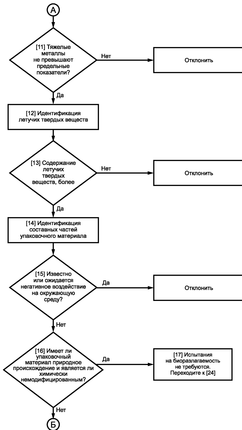
Рисунок В.1, лист 2
