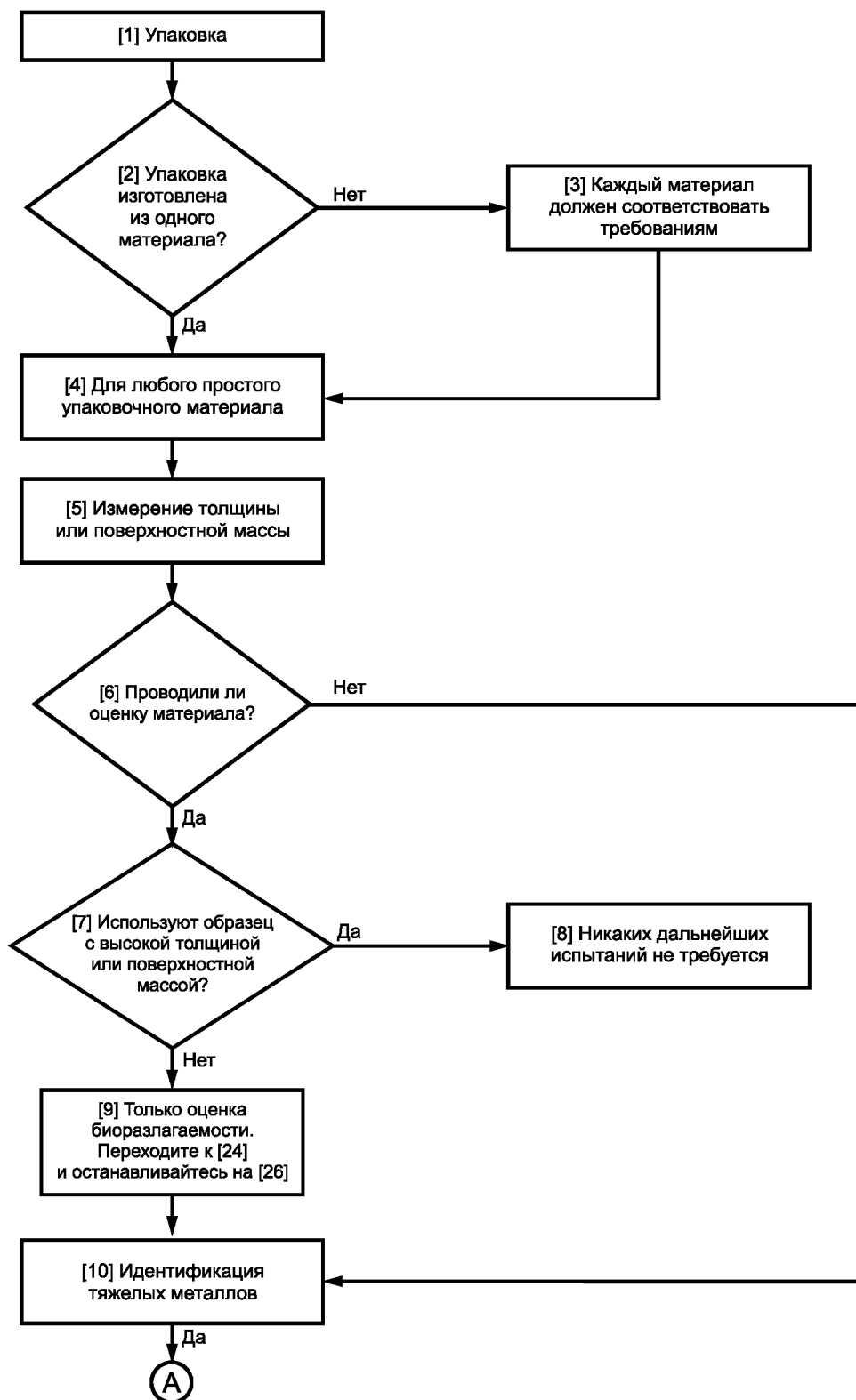
Рисунок В.1, лист 1
