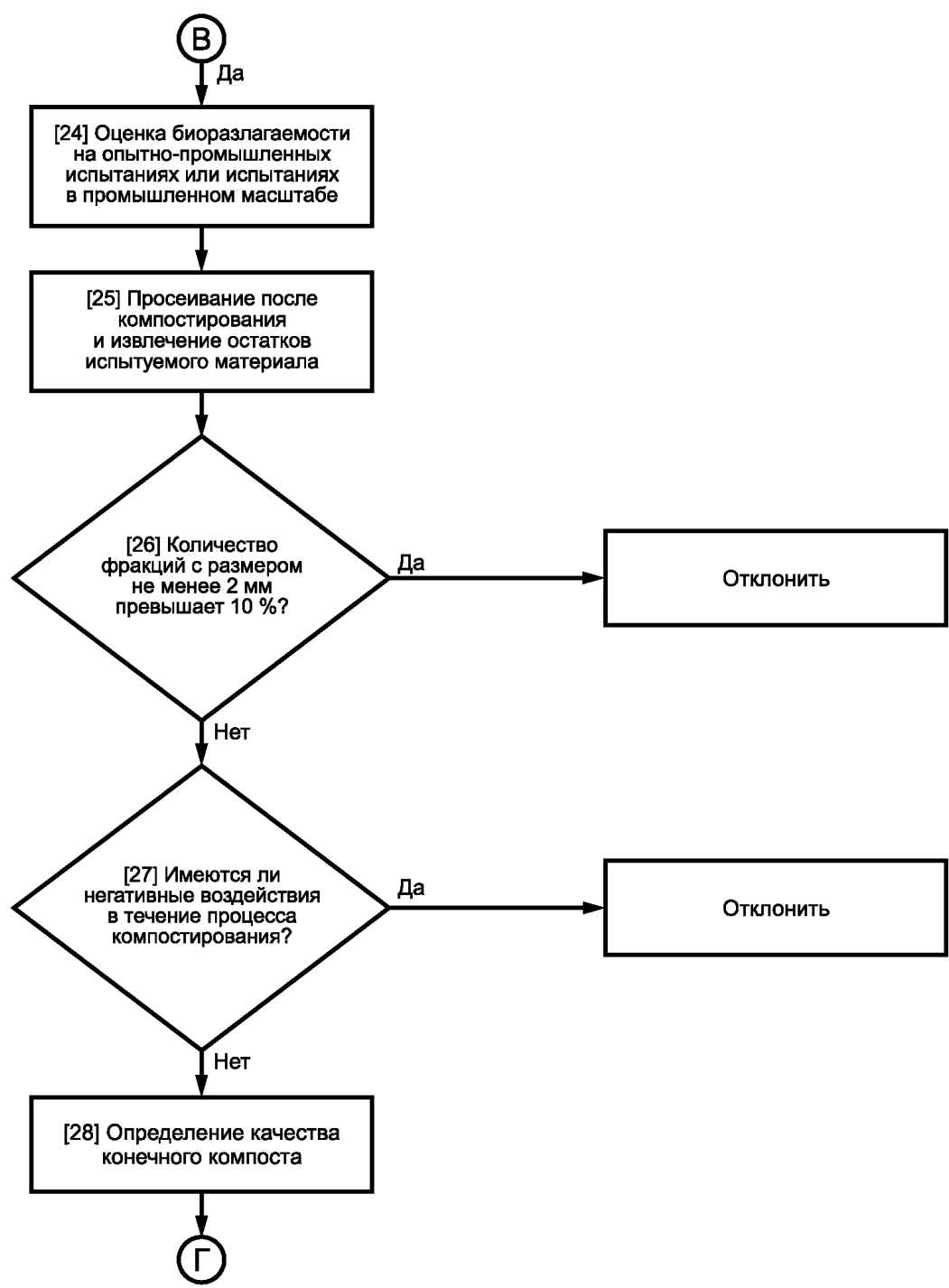
Рисунок В.1, лист 4
