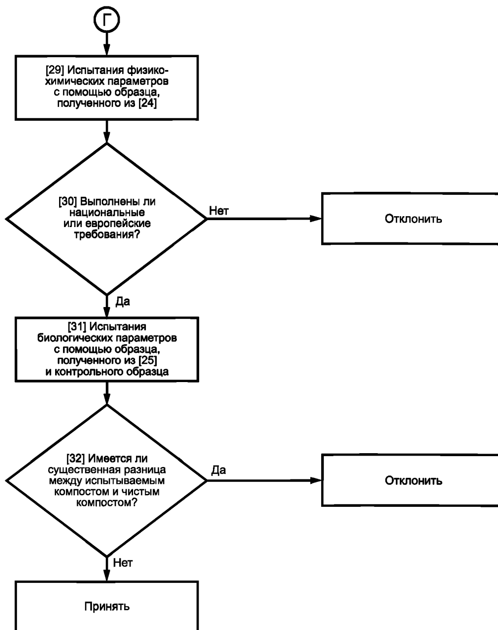
Рисунок В.1, лист 5
