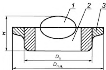
Рисунок 1 — Габаритные размеры ПКС
