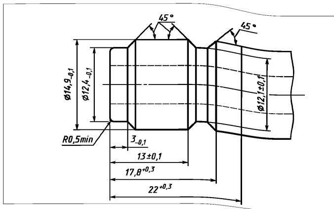
Рисунок 3 – Основные размеры входного и выходного соединителей полости по диализату
