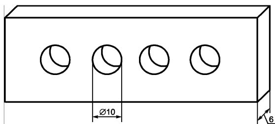
Рисунок 3 — Форма для образцов при испытании на текучесть
