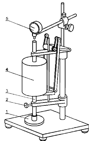
1 — латунная пластина; 2 — стопорный винт; 3 — вал; 4 — металлический цилиндр; 5 — датчик
