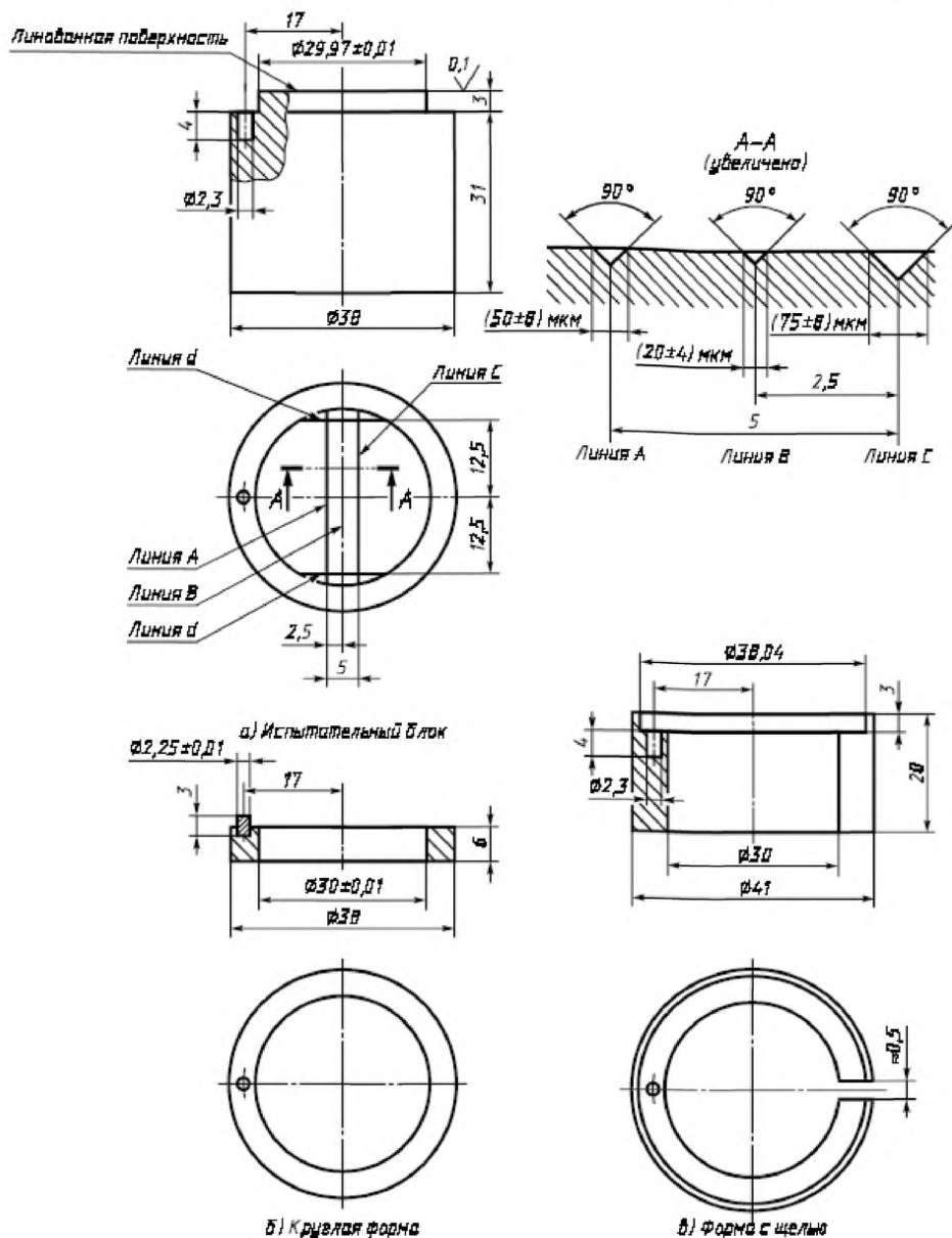
Рисунок 1 – Схема прибора для воспроизведения деталей
