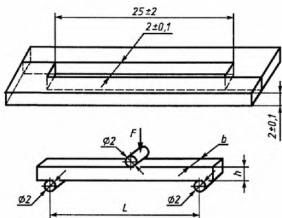
Рисунок 1 — Форма и приспособление для испытания на изгиб
