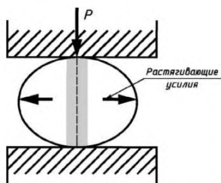
Рисунок 2 — Схема испытания на прочность при диаметральном разрыве
