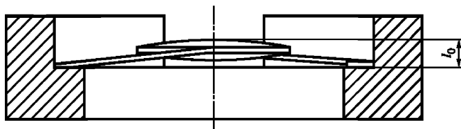
Рисунок Б.1 — Цилиндрический колодец с ИОЛ в несжатом состоянии
