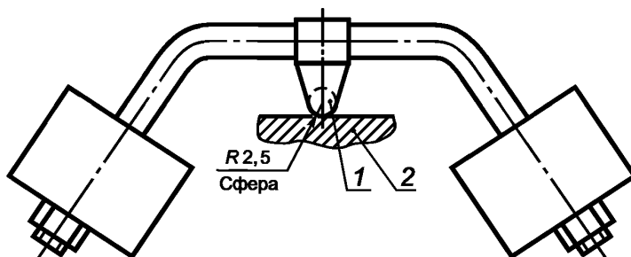
1 — стальной шарик диаметром 5 мм; 2 — образец
