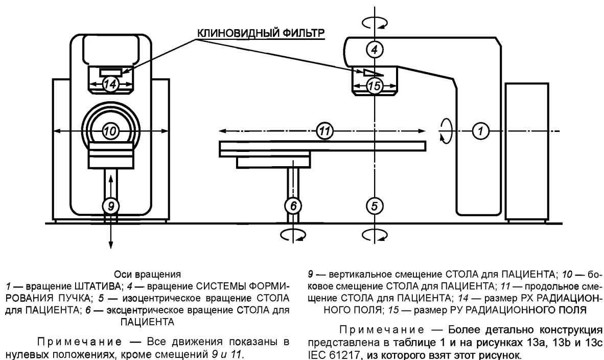
Рисунок 108 — Движение АППАРАТА и шкалы.
