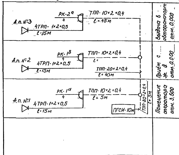
Скелетная схема громкоговорящей связи
