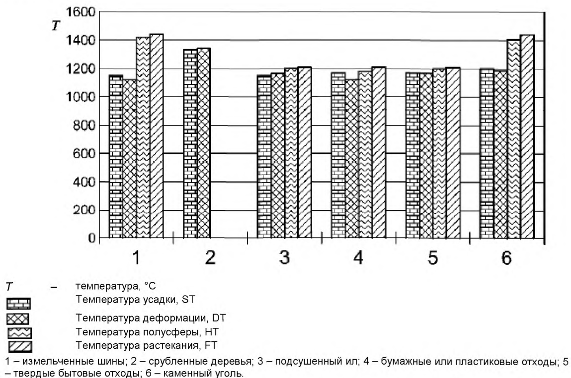
Рисунок 4 – Характерные температуры для твердого топлива из бытовых отходов
