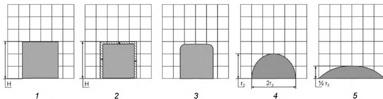
1 — исходный образец; 2 — усадка; 3 — деформация; 4 — полусфера; 5 — растекание.
