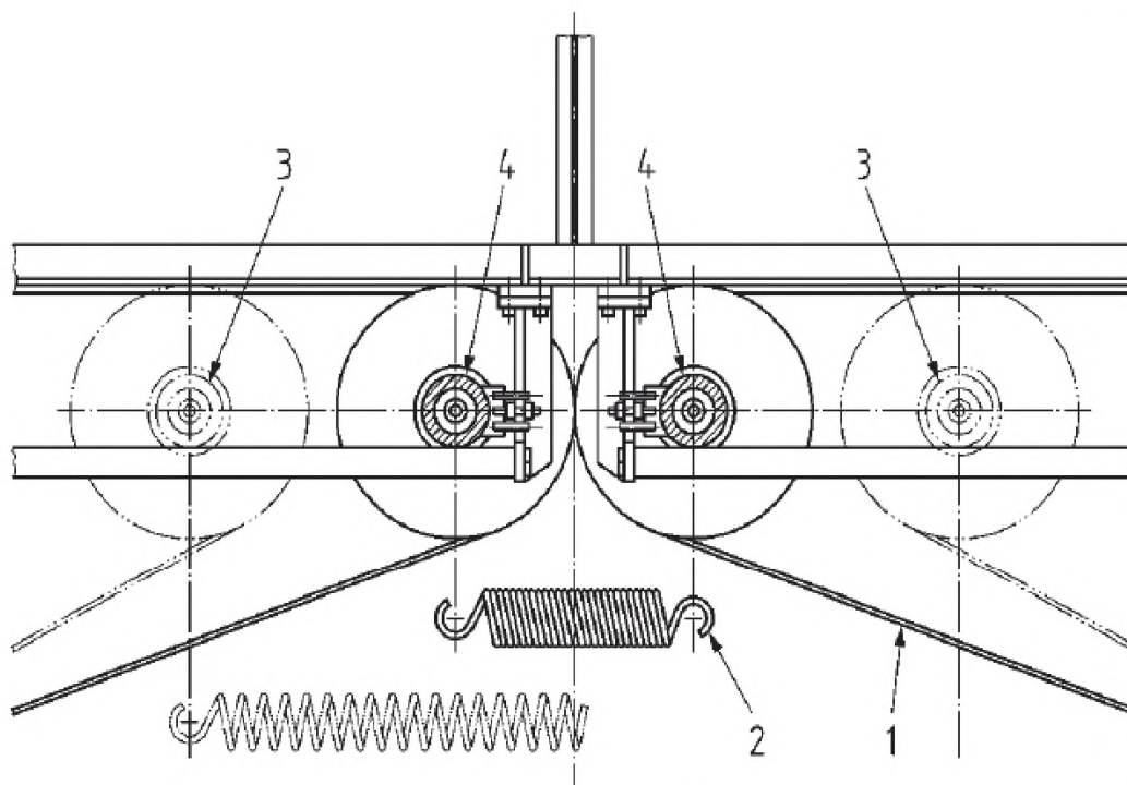
Рисунок 2 – Принцип работы аппарата для определения степени сводообразования сыпучего материала
