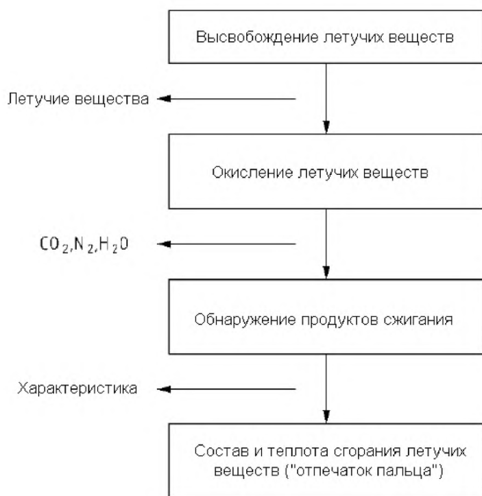
Рисунок 17 — Принцип измерений
