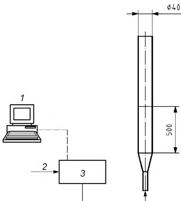
1 – регистратор данных; 2 – воздушный поток; 3 – поток материала
