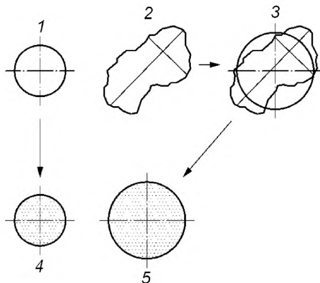
1 – круглый объект правильной формы; 2 – объект неправильной формы; 3 – круг с эквивалентной площадью поверхности; 4 – сфера с площадью проекции, равной площади круглого объекта; 5 – сфера с площадью проекции, равной площади объекта неправильной формы
