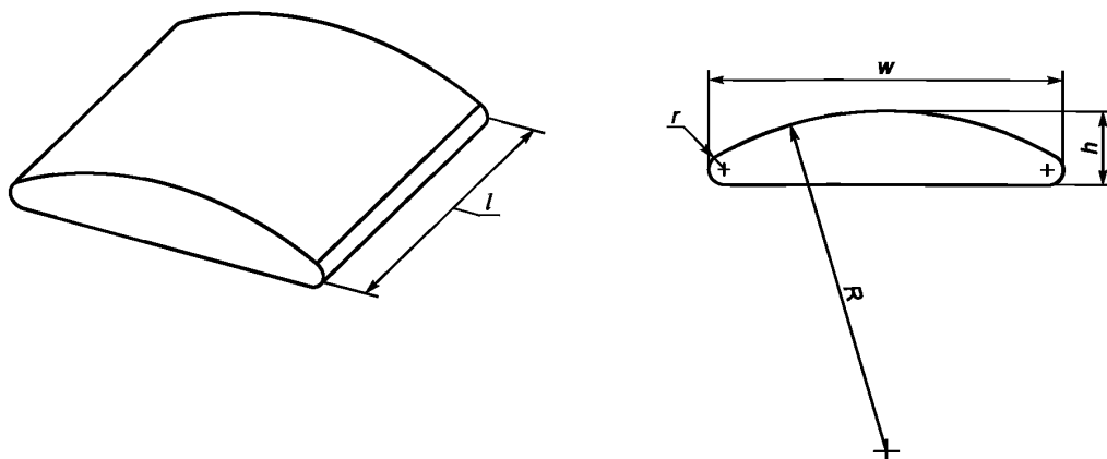
Рисунок 7 — Переменная выпуклая нагрузочная подушка
