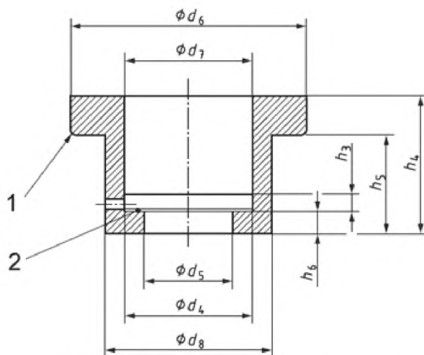
Рисунок А.3 – Промежуточное кольцо, тип В
