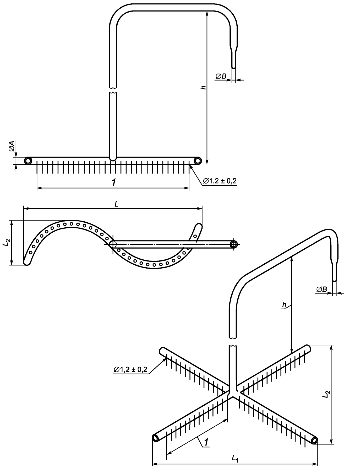
1 — подъем 15 мм; A — наружный диаметр 12 мм; B — наружный диаметр 8 мм; h — в зависимости от высоты пробоотборника; L, L 1 и L 2 — в зависимости от положения вывода газа; материал — нержавеющая сталь Рисунок 6 — Зонд отбора проб для газовых аппаратов типов А и В с дымовой трубой
