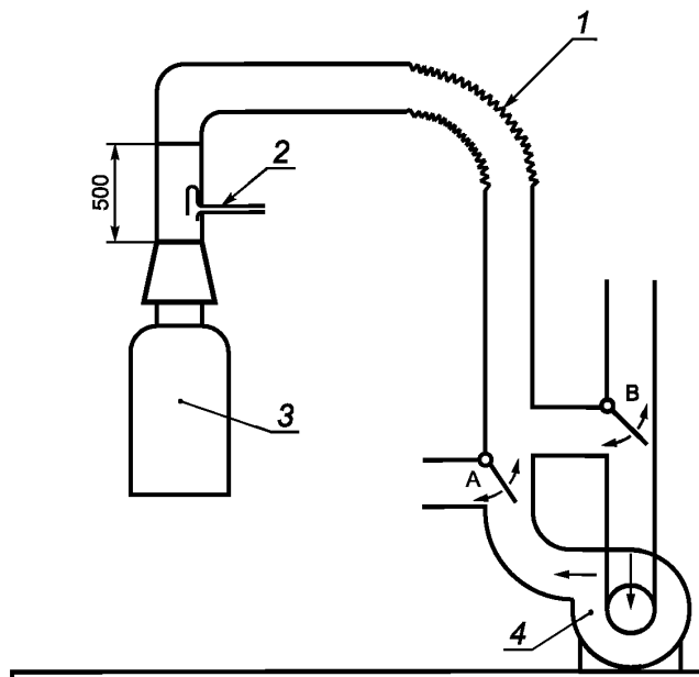
А и В — переборки для получения прямой и обратной тяги; 1 — гибкая труба; 2 — место для измерения скорости с помощью трубки Пито; 3 — аппарат; 4 — вентилатор
