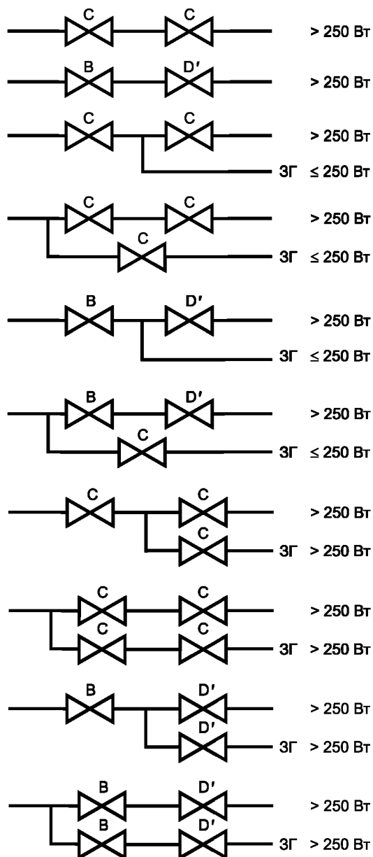
Рисунок В.2. ЗГ — запальная горелка
