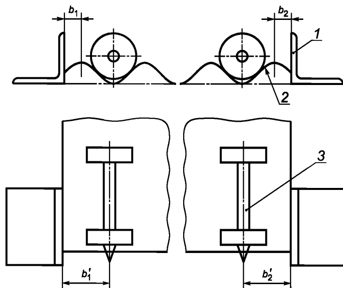
1 — металлический упор; 2 — лист; 3 — металлический цилиндр
