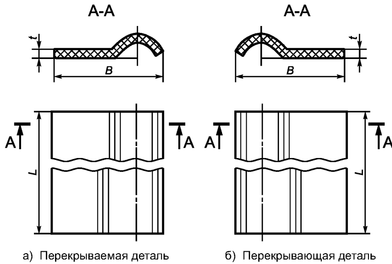
Рисунок 8 — Упрощенные коньковые детали
