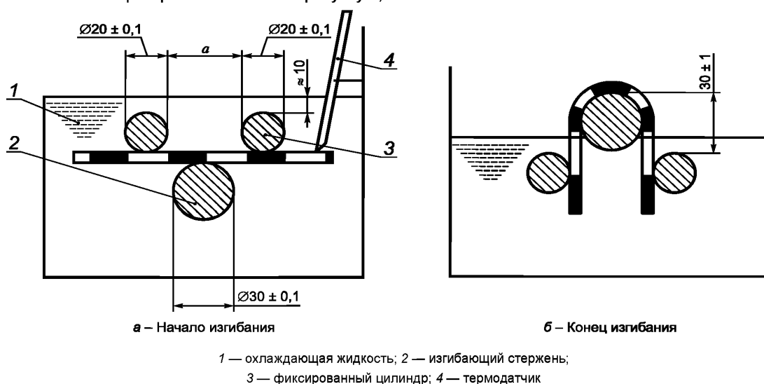
Рисунок 1 — Конструкция и принцип действия изгибающего приспособления
