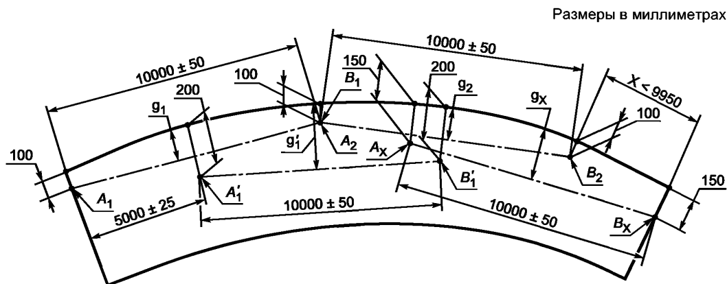
Рисунок 2 — Пример схемы нанесения контрольных линий на полотно материала, длина которого превышает 10,05 м
