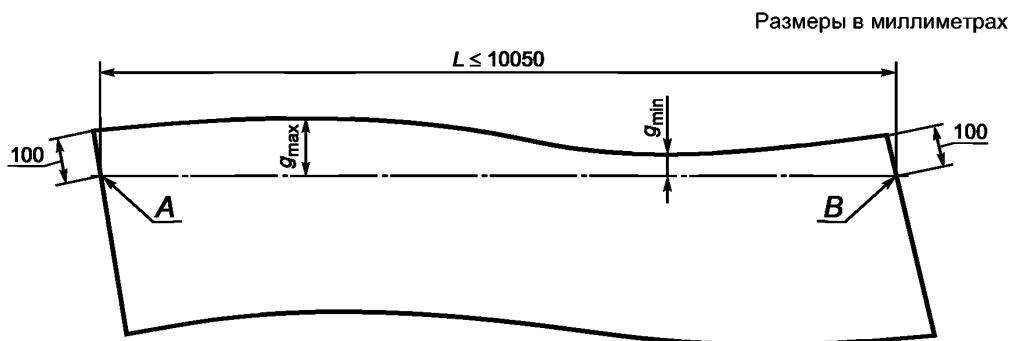
Рисунок 1 — Схема нанесения контрольной линии на полотно материала, длина которого не превышает 10,05 м
