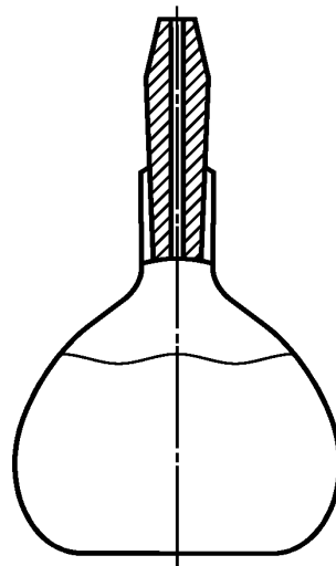
Рисунок 2 — Стекланный пикнометр типа Гей-Люссака
