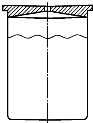
Рисунок 1 — Металлический пикнометр
