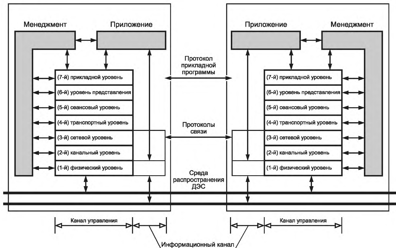
Рисунок А.10 — Общее представление эталонной модели ДЭС
