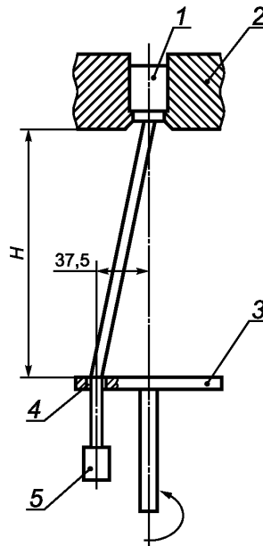
Рисунок 101 — Устройство для испытания прочности изоляции проводников
