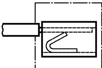
Безвинтовой зажимной элемент с прямым зажимом
