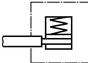
Безвинтовой зажимной элемент с непрямым зажимом
