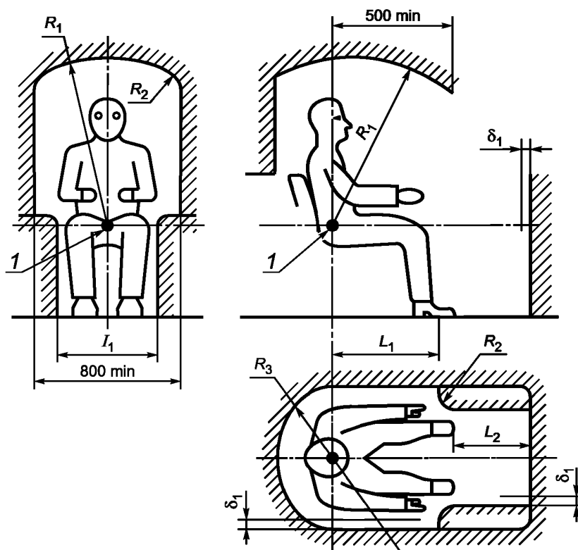
Рисунок 4 — Размеры кабины
