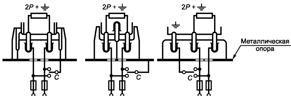
Рисунок 8 — Схемы соединения для испытания на нормальную работу
