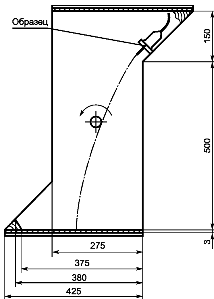
Рисунок 11 — Барабан для испытания соединителей на свободное падение
