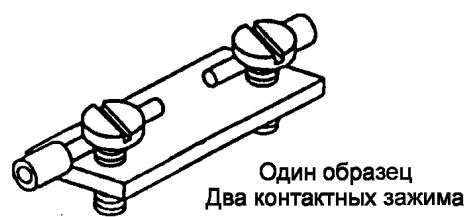
Рисунок F.1 — Непосредственный зажим головкой винта неподготовленных проводников
