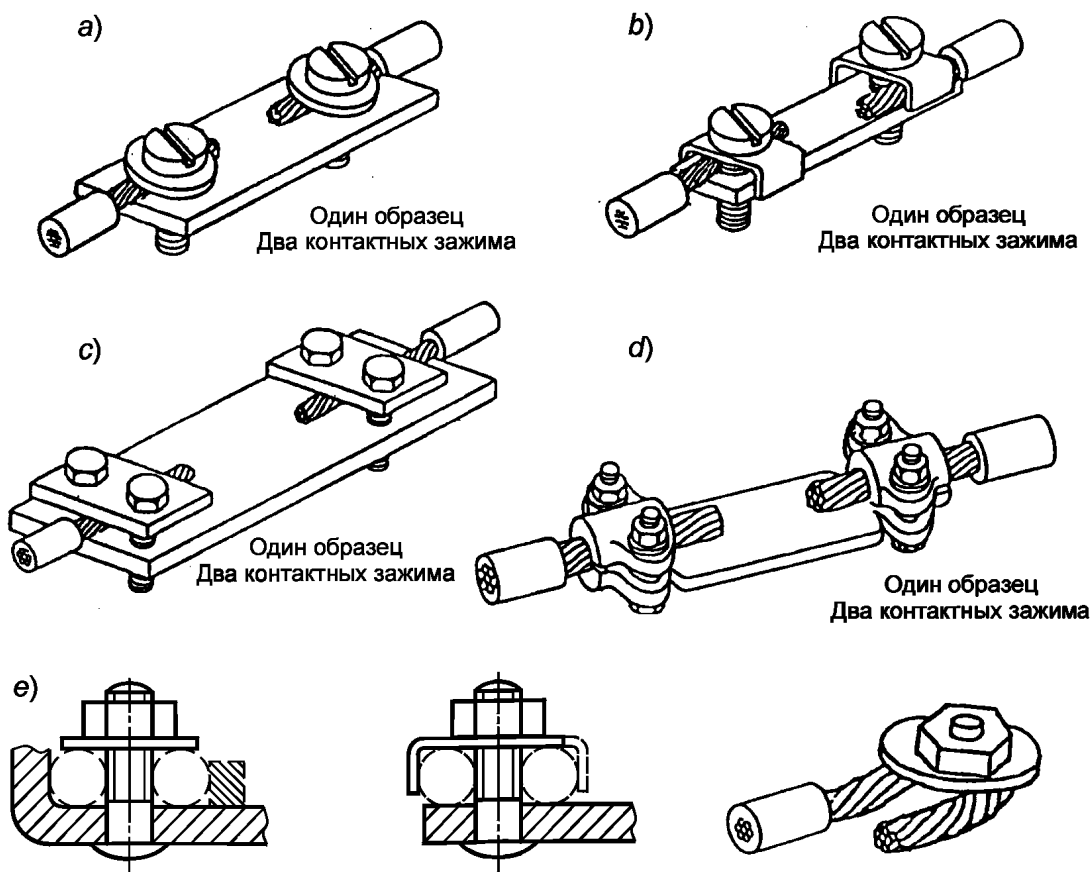
Рисунок F.2 — Косвенный зажим с помощью промежуточной детали неподготовленных проводников
