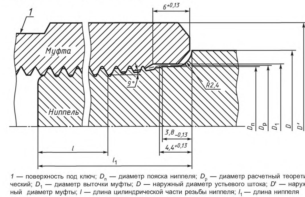
Рисунок 12 — Сопрягаемые элементы ниппелей устьевых штоков и муфт для них
