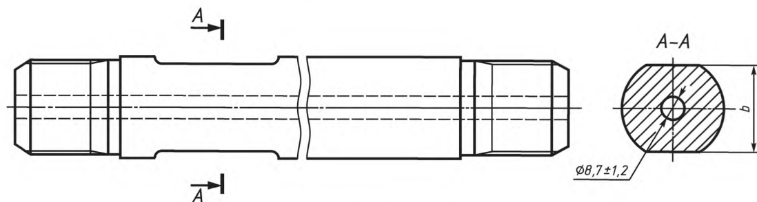
б — устьевой шток полый
