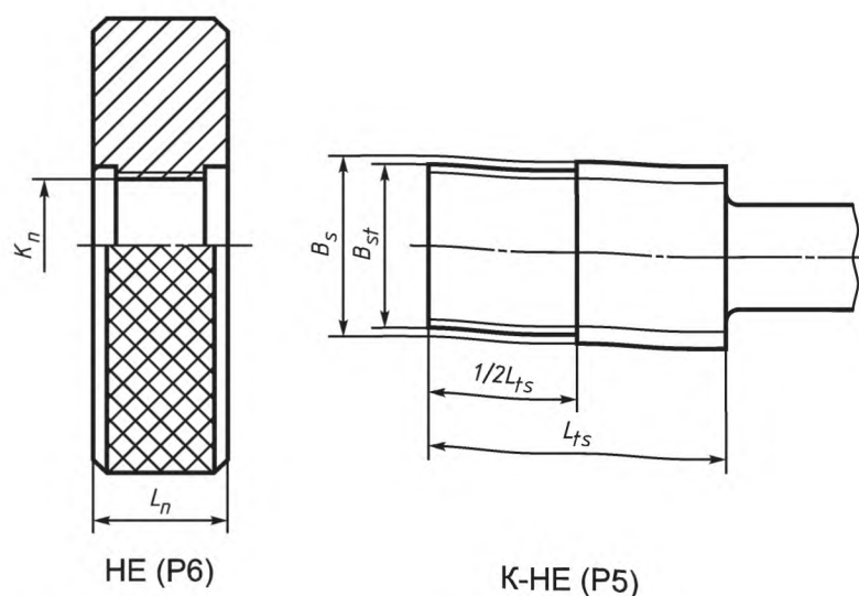
Рисунок Д.2 — Основные размеры калибров НЕ (P6) и К-НЕ (P5) для контроля резьбы ниппеля
