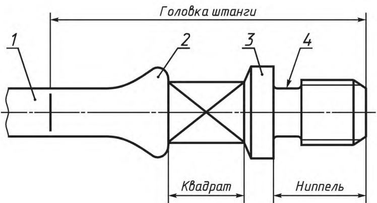
1 — тело штанги; 2 — подэлементарный бурт; 3 — упорный бурт; 4 — резьбовая канавка
