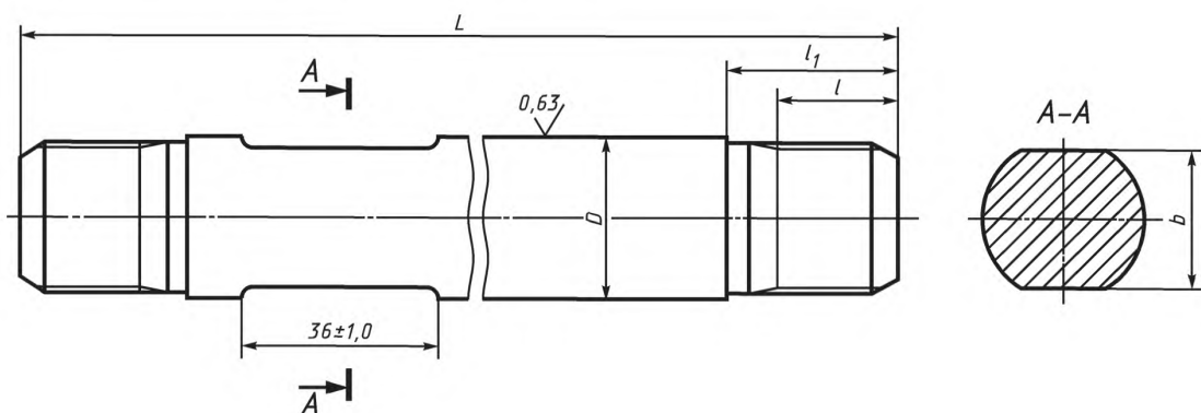
а — устьевой шток цельный
