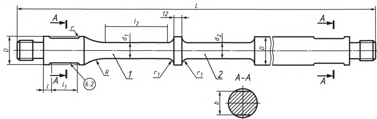
Рисунок 8 — Утяжеленная штанга
