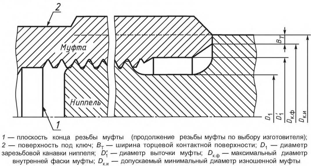
Рисунок 11 — Сопрягаемые элементы ниппелей штанг и муфт к ним
