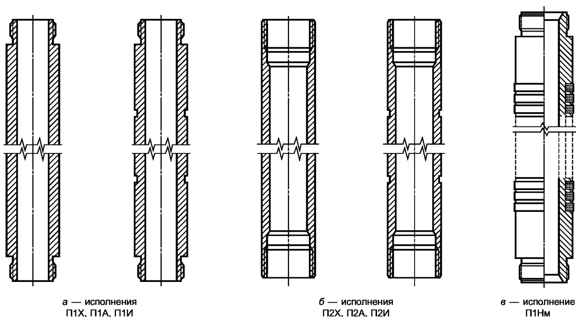
Рисунок 15 — Плунжеры
