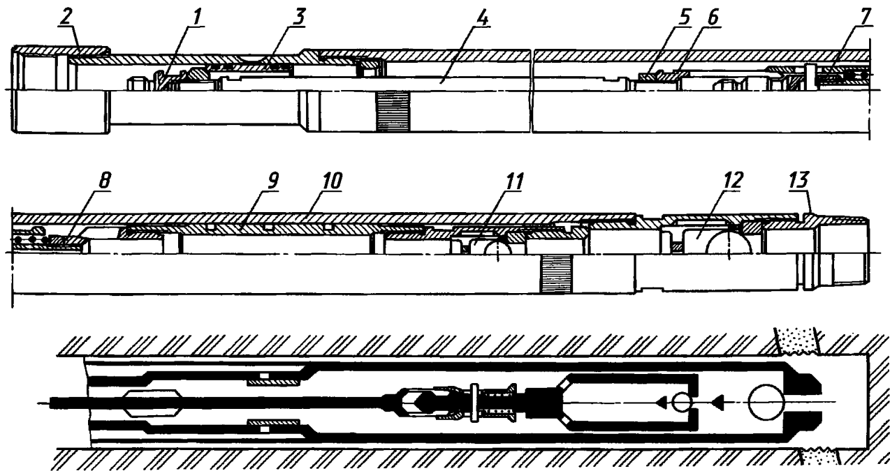
1 — переводник штока; 2 — верхний переводник; 3 — сливное устройство; 4 — шток; 5 — контргайка; 6 — цанговый захват; 7 — сцепляющее устройство; 8 — переводник плунжера; 9 — плунжер; 10 — цилиндр; 11 — нагнетательный клапан; 12 — всасывающий клапан; 13 — переводник насоса
