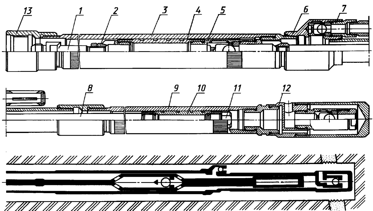
1, 8 — штоки; 2 — переводник плунжера; 3 — цилиндр насоса; 4, 10 — плунжеры; 5 — нагнетательный клапан; 6 — клапанный блок; 7 — всасывающий клапан; 9 — цилиндр гидроусилителя; 11 — наконечник; 12 — разрядный клапан; 13 — переводник насоса
