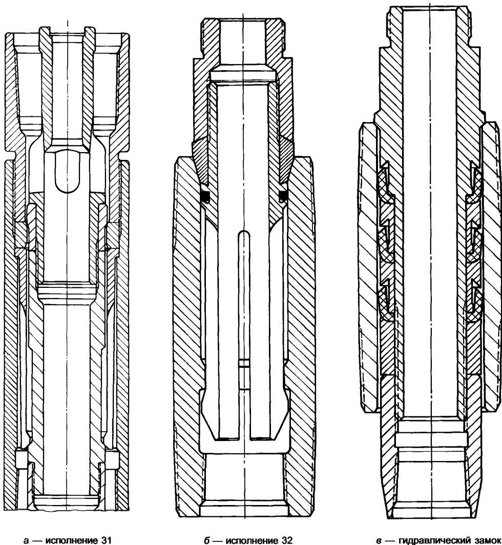
Рисунок 17 — Замки
