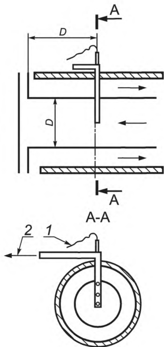
1 — к датчику температуры; 2 — к насосу пробоотборника
