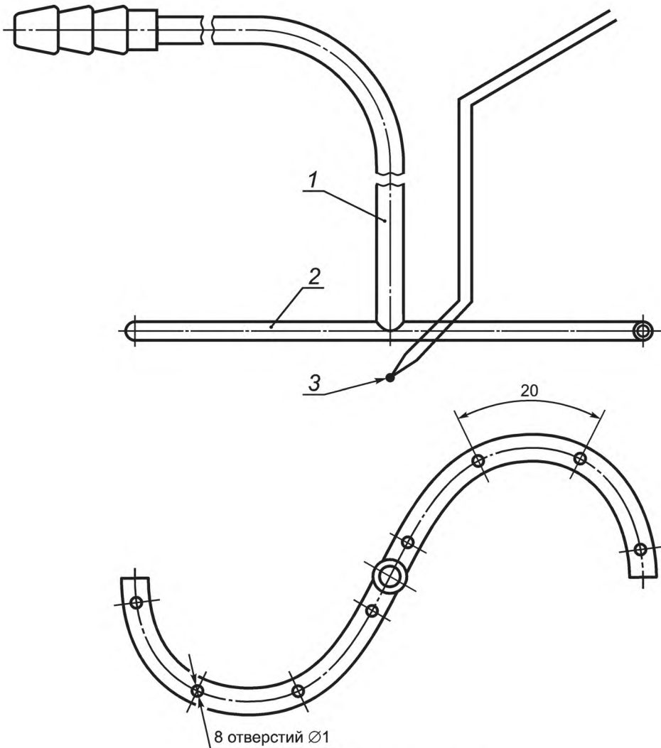
1 — медная трубка Ø 6 мм; 2 — медная трубка Ø 4,3 мм; 3 — термопара Рисунок 10 — Пробоотборник для отбора проб продуктов сгорания для испытательных дымоходов диаметром D < 100 мм
