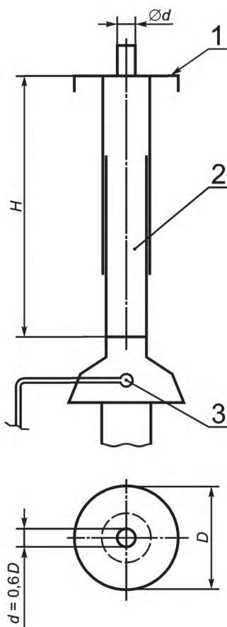
1 — пластина; 2 — телескопический испытательный дымоход; 3 — детектор
