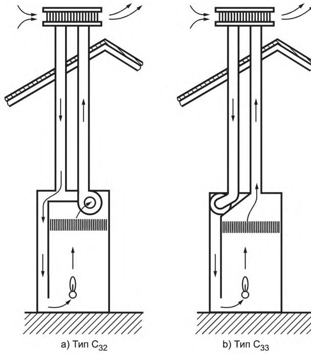
Рисунок В.3 — Водонагреватели типа C 3
