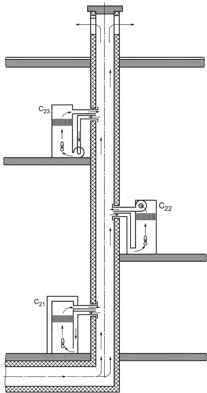
Рисунок В.2 — Водонагреватели типа C 2
