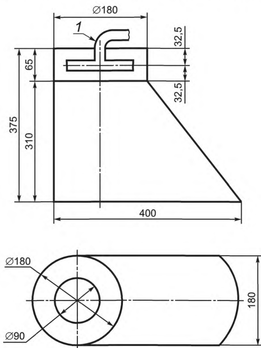
1 — пробоотборник (рисунок 7)
