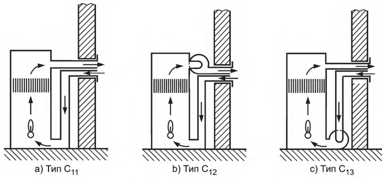
Рисунок В.1 — Водонагреватели типа С 1
