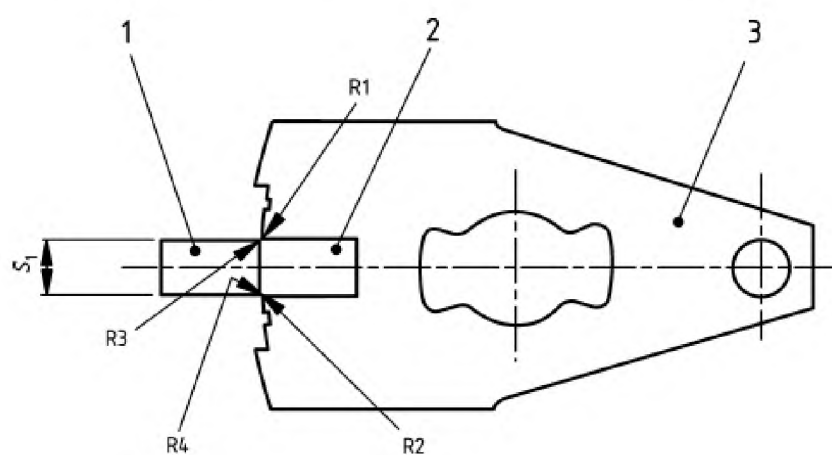
1— стопорный элемент; 2 — кодовый канал; 3 — сувальда
