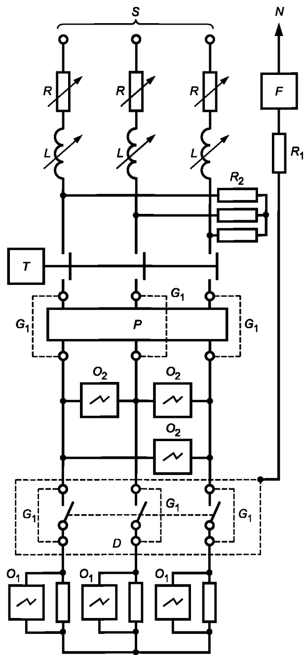
S – источник питания; R – регулируемый резистор нагрузки; L – регулируемая катушка индуктивности нагрузки; T – замыкающее устройство; F – медный проволочный предохранитель; R_1 – резистор ограничения тока повреждения; R_2 – резистор, отводящий ток 10 А на фазу; P – УЗКЗ; G_1 – временное калибровочное соединение; O_1 – датчик тока; O_2 – датчик напряжения; D – испытуемый выключатель-разъединитель
