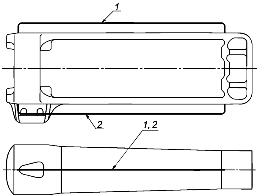
Рисунок В.2 — Схема разметки кернами тягового хомута
