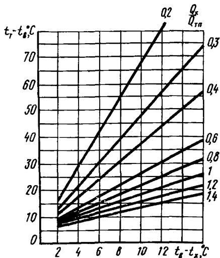
Рис. 8. Зависимость температуры теплоносителя от температуры хладагента и соотношения холодо- и теплонагрузок для радиационных систем
