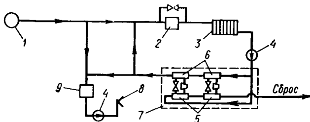
Рис. 19. Схема с применением пикового подогрева и тепловых насосов 1 — скважина; 2 — пиковая котельная; 3 — система отопления; 4 — насос; 5 — испарители; 6 — конденсаторы; 7 — теплонасосная установка; 8 — система горячего водоснабжения; 9 — бак-аккумулятор
