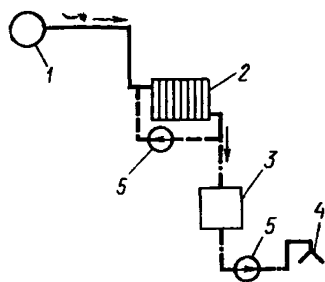
Рис. 14. Схема с последовательной подачей геотермальной воды на отопление и горячее водоснабжение
