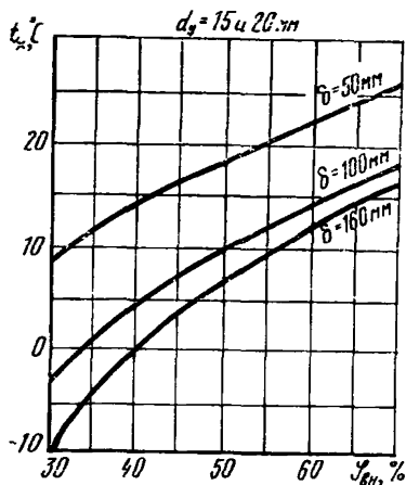
Рис. 6. Зависимость температуры теплоносителя t_x от относительной влажности внутреннего воздуха \Phi_{вн}
