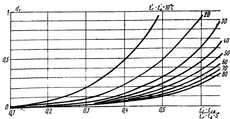
Рис. 2. Доля пикового обогрева при отоплении
