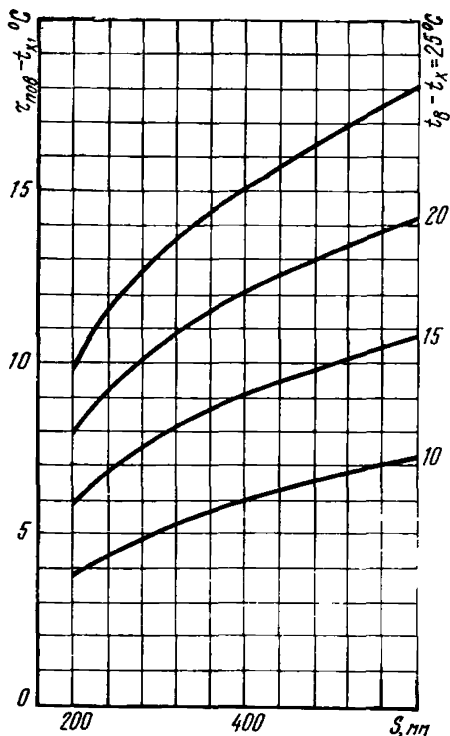
Рис. 8. Зависимость температуры теплоносителя от температуры хладагента и соотношения холодо- и теплонагрузок для радиационных систем
