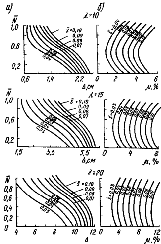
Рис. 15. Графики зависимости между \bar{N} , \bar{S} и \mu (а) и \bar{N} , \bar{S} и \lambda (б) при гибкости колонны \lambda = 10, 15, 20 и упругой работе арматуры
