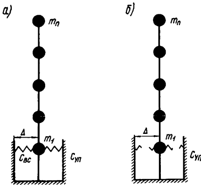
Рис.1. Расчетные схемы зданий с выключающимися связями
