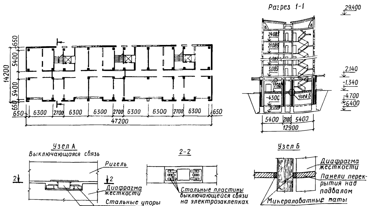
Рис.10. Крупнопанельное здание на железобетонных стойках в первых двух этажах с выключающимися связями и диафрагмами жесткости (проект разработан Таджикгипростроем совместно с ЦНИИСК им.В.А.Кучеренко)
