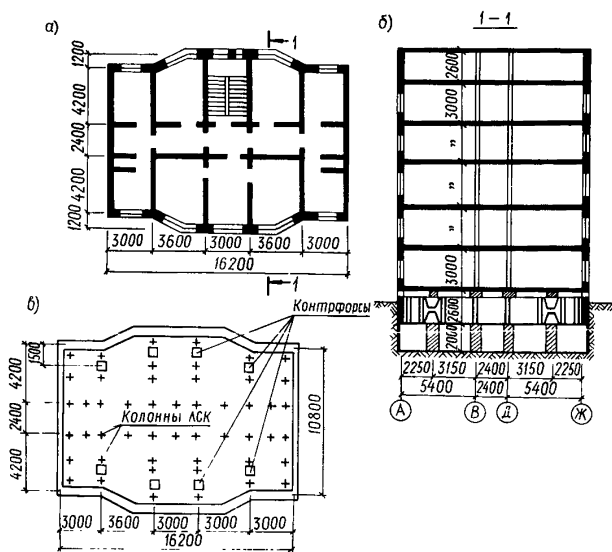
Рис.6. Конструктивное решение крупнопанельного дома серии 122 с выключающимися связями а - план рядовой блок-секции; б - разрез; в - план рядовой блок-секции на отметке 0,90 м
