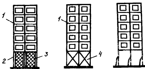
Рис. 5. Здания с выключающимися связями в нижних каркасных этажах
