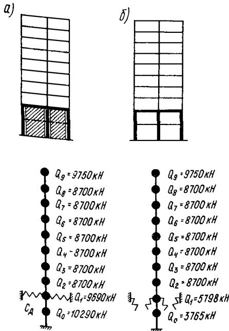
Рис.14. Расчетные модели 9-этажного здания на железобетонных стойках с выключаемыми диафрагмами в состоянии до выключения (а) и после выключения (б) диафрагм
