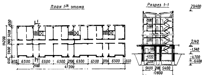
Рис. 13. Крупнопанельное здание на железобетонных стойках с выключающимися диафрагмами
