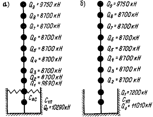
Рис.11. Расчетные модели 9-этажного здания в состоянии до выключения (а) и после выключения (б) связей
