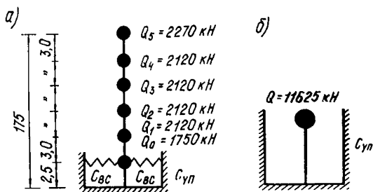
Рис. 7. Расчетные модели здания в состоянии до выключения (а) и после выключения (б) связей
