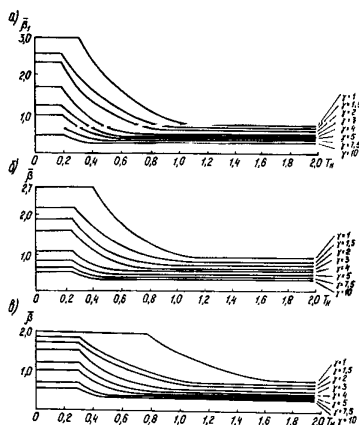
Рис. 2. Графики определения расчетных значений динамического коэффициента для зданий с выключающимися связями в зависимости от категорий грунтов по сейсмическим свойствам
