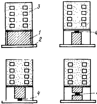
Рис. 3. Конструктивные решения зданий с нижним гибким этажом и с выключающимися связями
