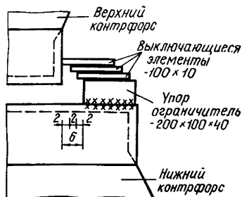
Рис. 8. Конструирование элементов выключающейся связи
