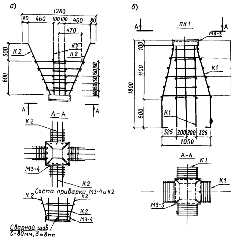
Рис. 9. Схемы армирования верхнего (а) и нижнего (б) контрфорсов в 5-этажном крупнопанельном здании серии 122 с ВС
