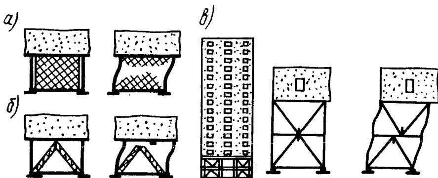
Рис.4. Конструктивные решения зданий с выключающимися связями
